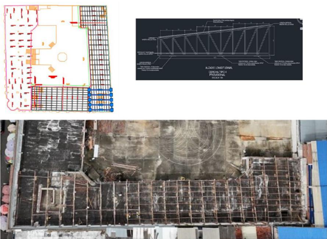
Figura 2- Suministro e instalación de cercha y correas tipo 4 para cubierta en madera rolliza inmunizada \phi=10 cm
