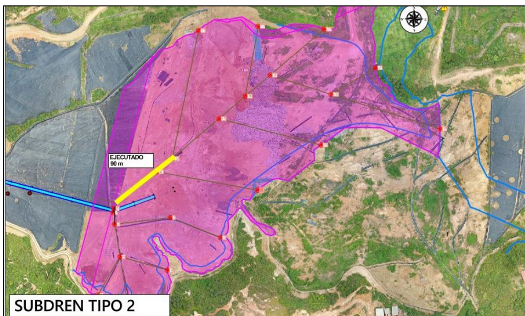
Figura. Localización subdrén de lixiviados construido
