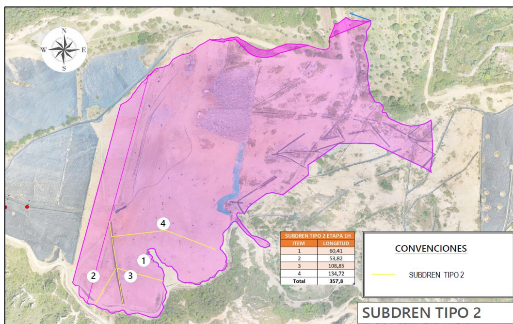
Figura. Subdrenes tipo 2 construidos
