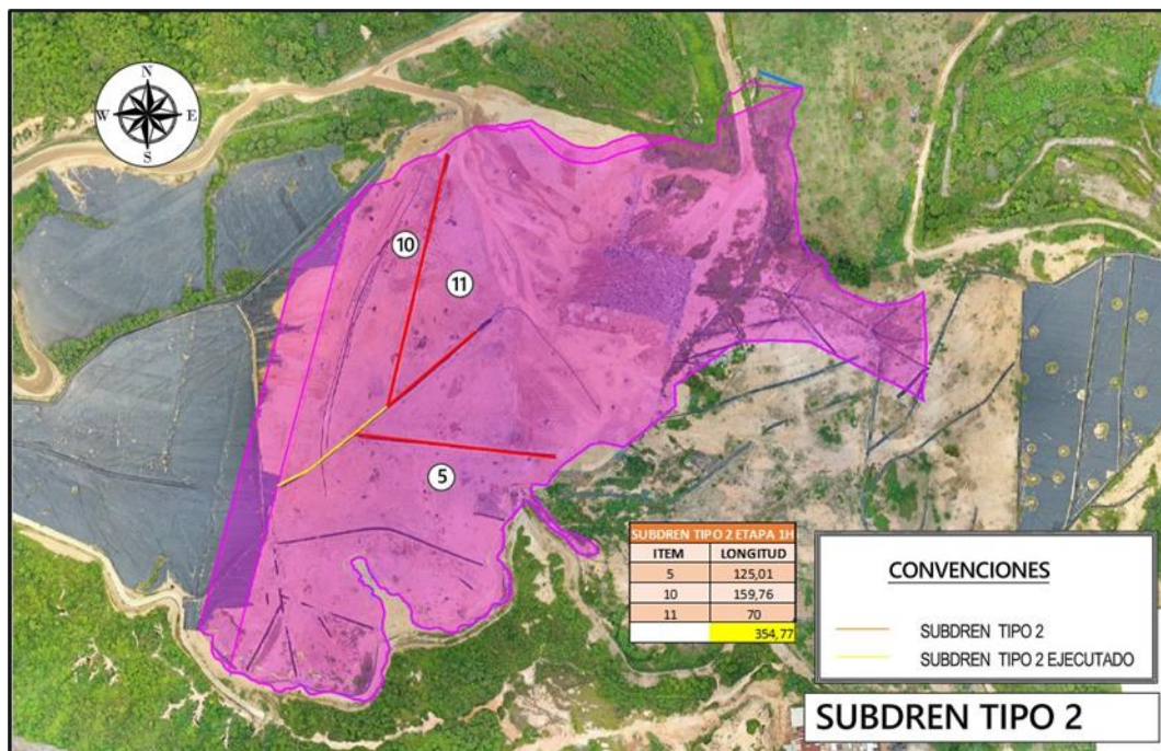
Figura. Localización subdrén de lixiviados construido mes de abril de 2026
