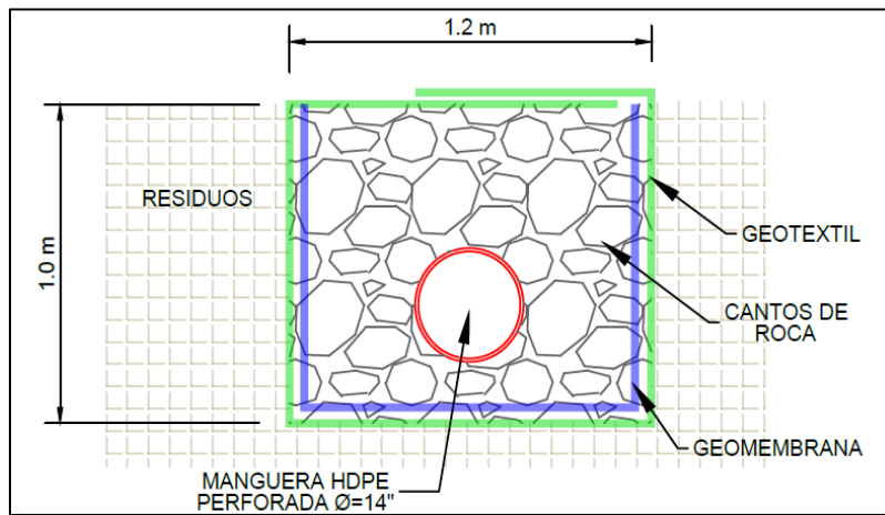
Figura. Esquema constructivo subdrén de lixiviados tipo 2
