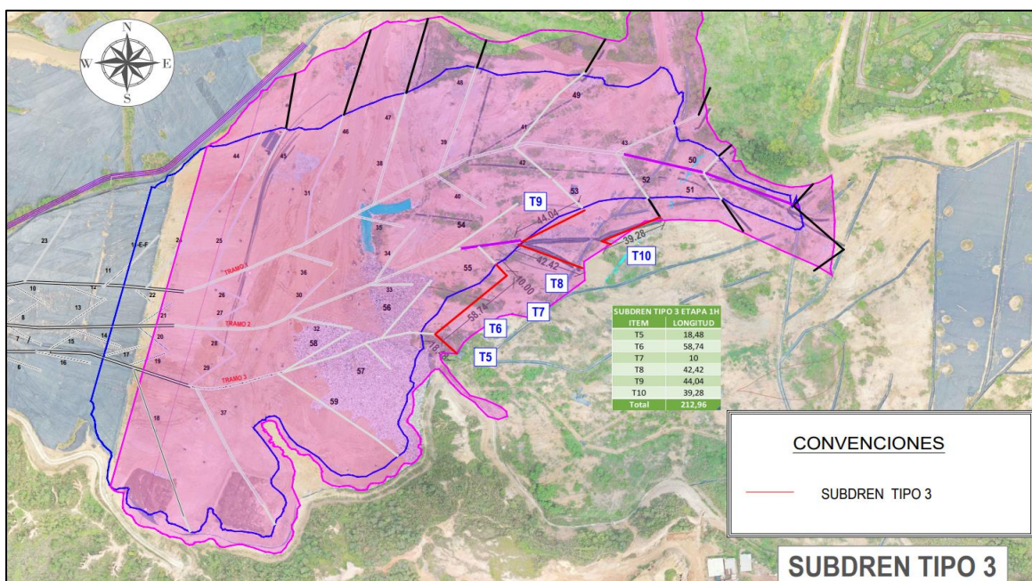
Figura. Subdrenes tipo 3 construidos
