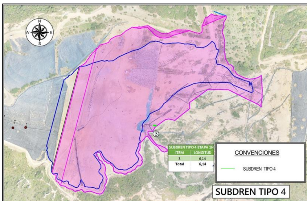
Figura. Subdrenes tipo 4 construidos
