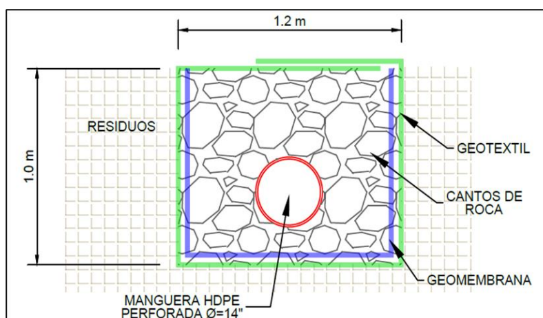
Figura. Esquema constructivo subdrén de lixiviados tipo 2
