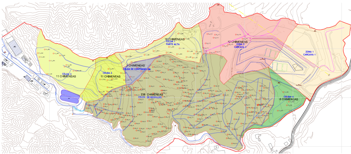
Figura. Chimeneas en el Sitio de Disposición Final El Carrasco.
