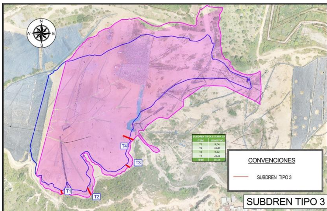
Figura. Subdrenes tipo 3 construidos
