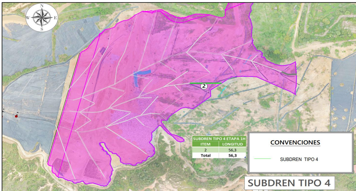
Figura. Subdrén tipo 4 construido
