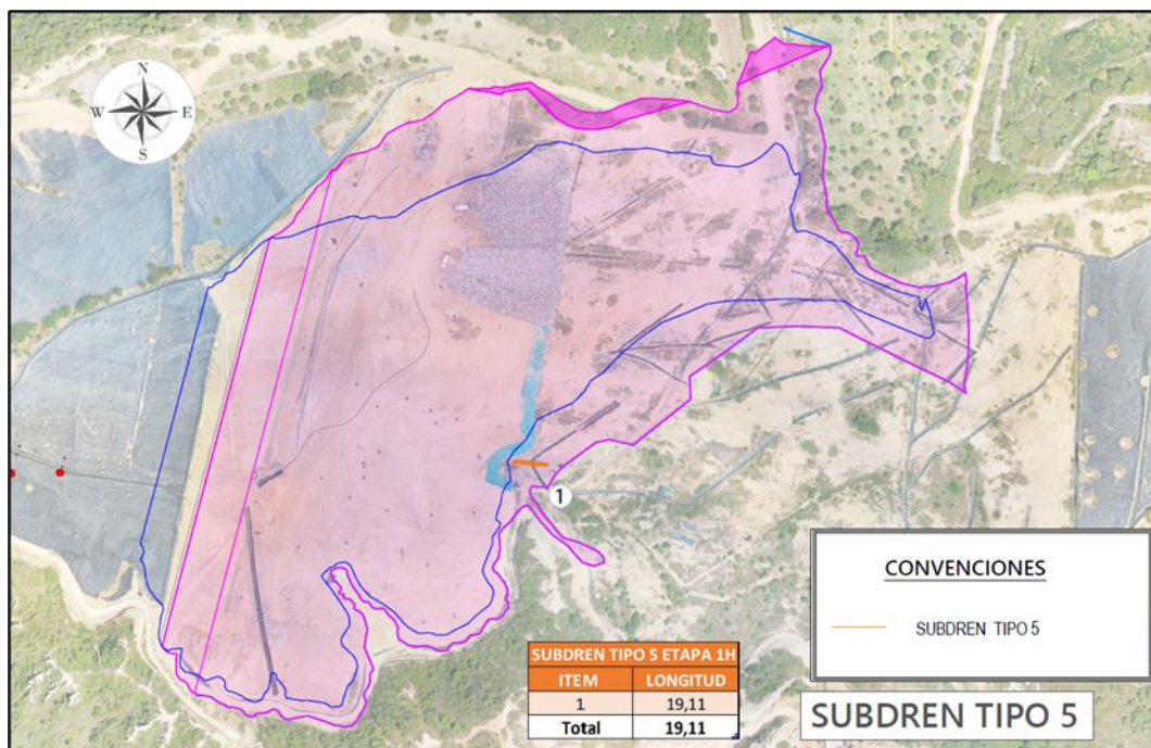
Figura. Subdrenes tipo 5 construidos
