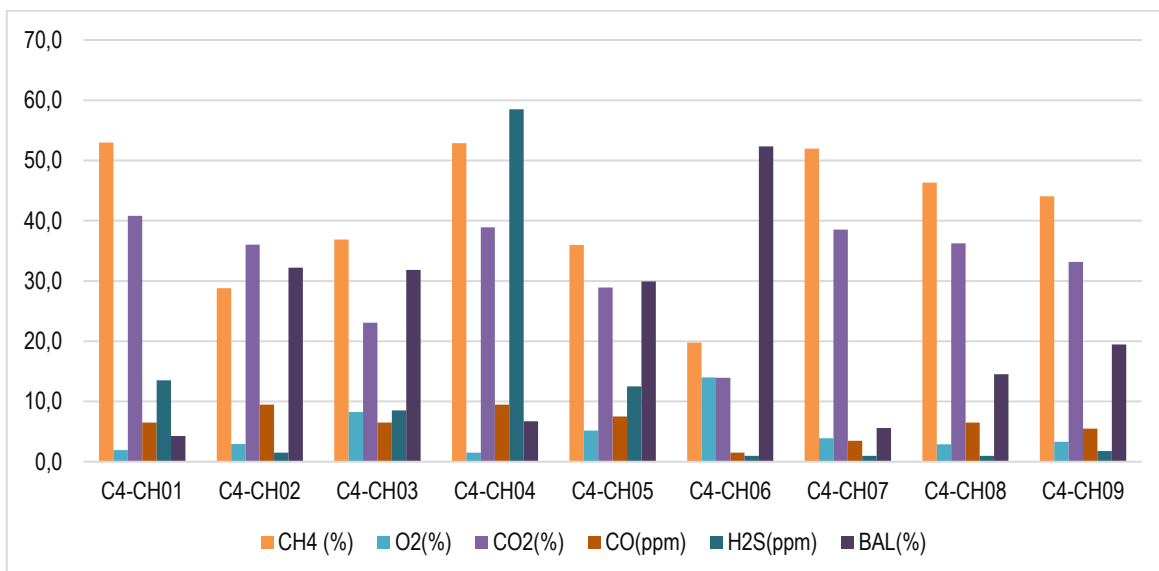
Gráfico 15 Caracterización de biogás celda de 4
