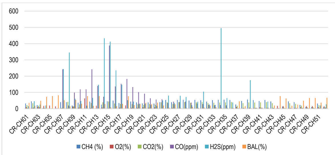
Gráfico 16 Caracterización de biogás celda de respaldo 1.
