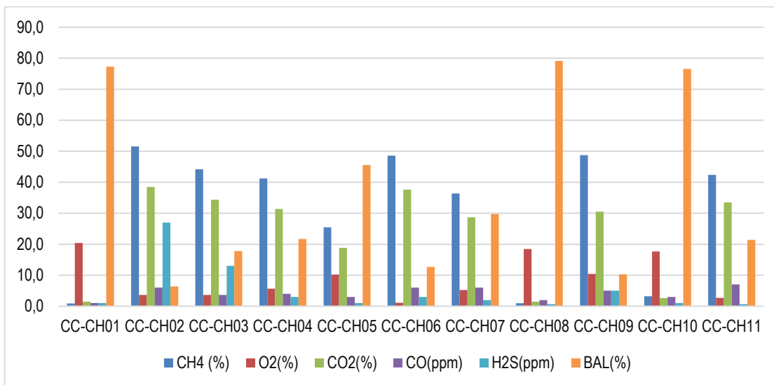
Gráfico 12 Caracterización de biogás celda de contingencia
