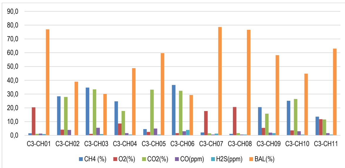
Gráfico 14 Caracterización de biogás celda de 3.
