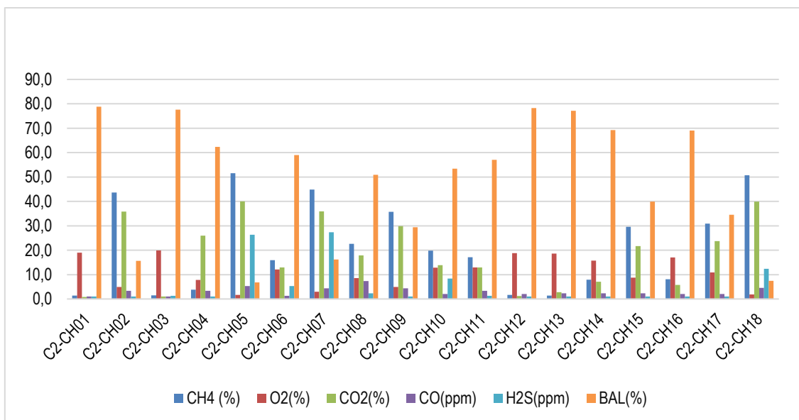
Gráfico 13 Caracterización de biogás celda 2.
