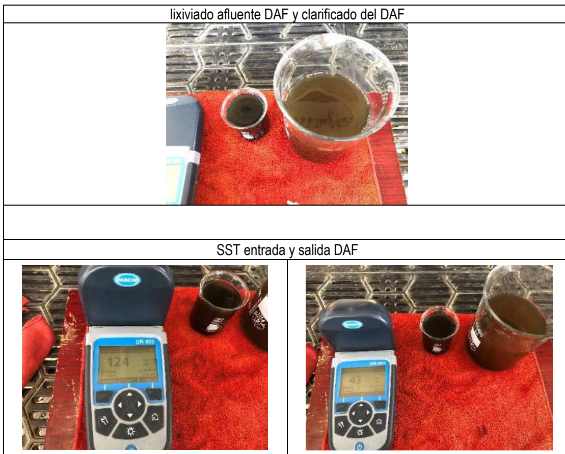
Ilustración 21 Medición de sólidos suspendidos totales (SST) en la entrada y salida DAF Apariencia
