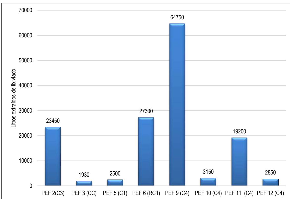
Gráfico 18 Volumen extraído de lixiviado primer trimestre 2021
