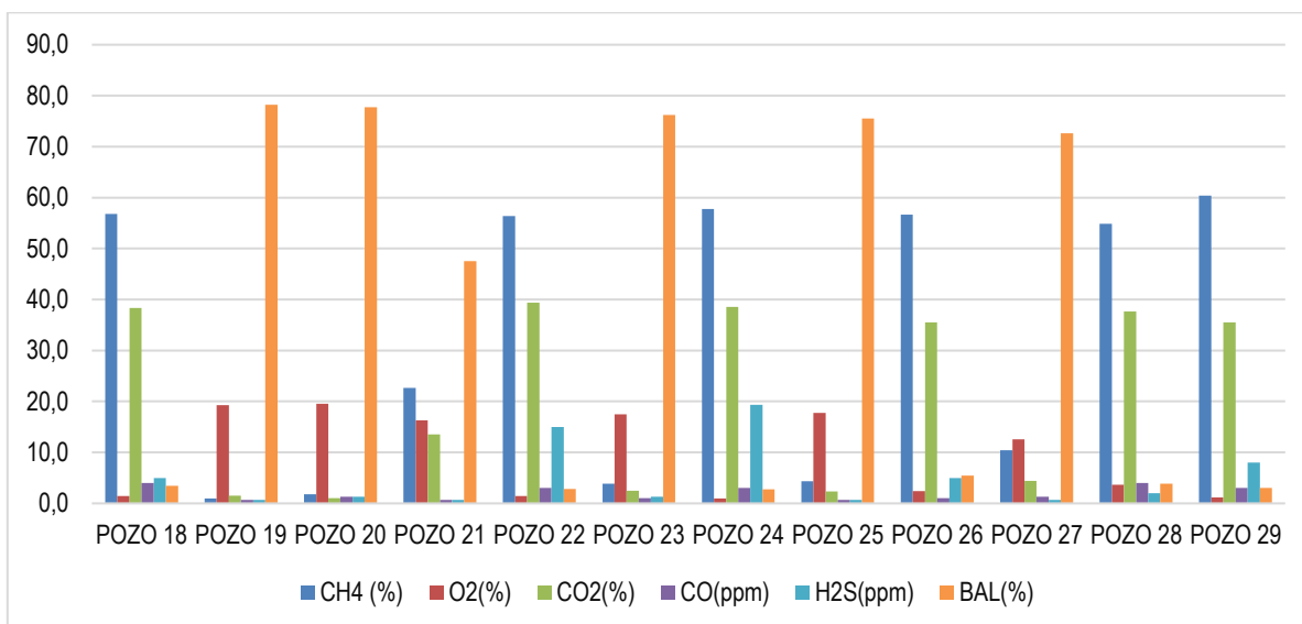
Gráfico 17 Caracterización de biogás zona clausurada.
