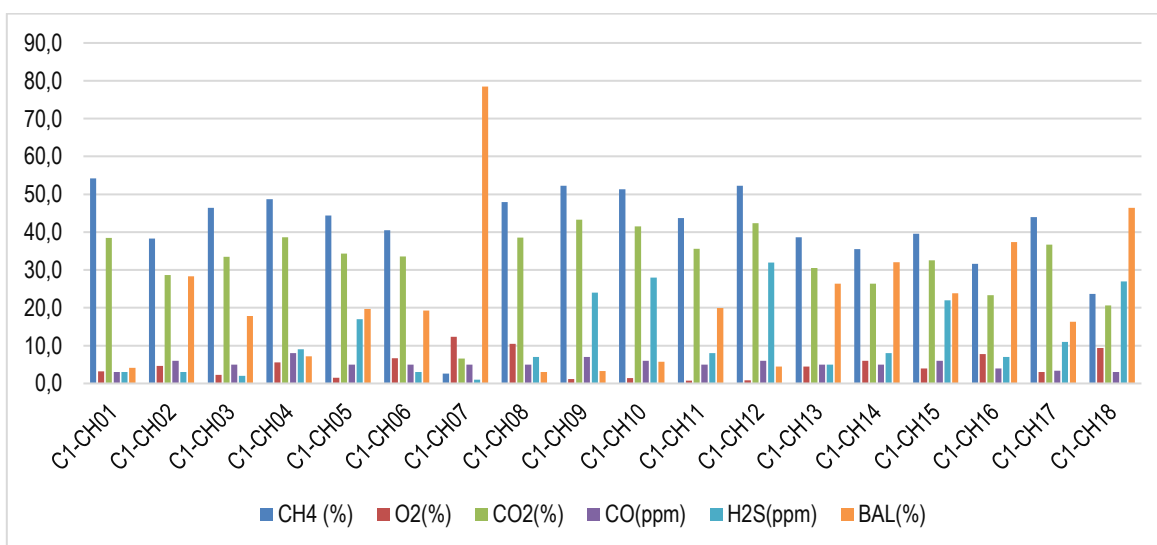
Gráfico 11 Caracterización de biogás celda 1.
